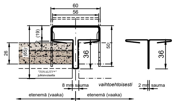
Saumaprofiili "SA"
