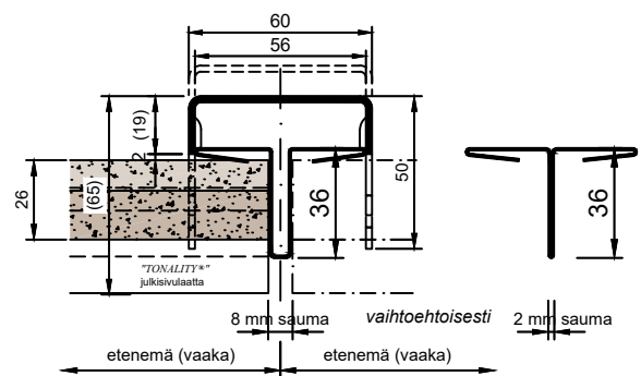
Saumaprofiili "SA"
