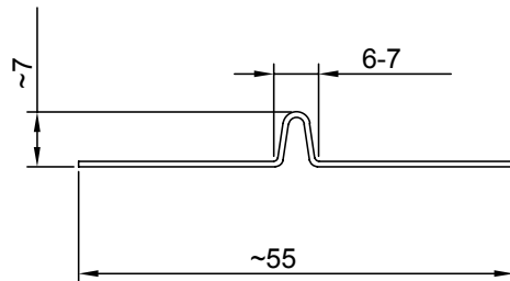
Saumalista omega
