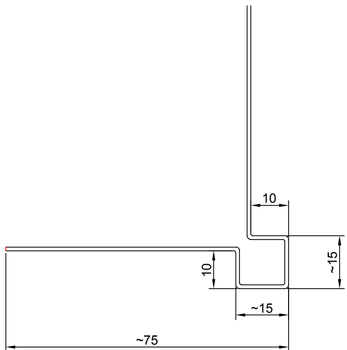
Ulkokulmalista
