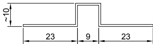
Pystysaumalista
