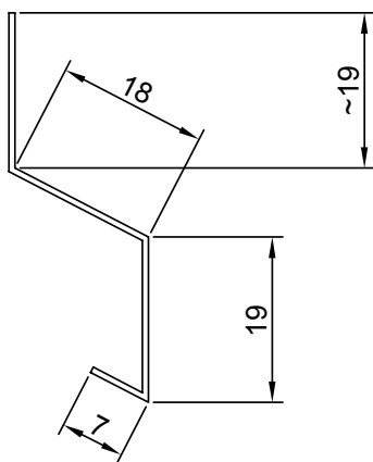
Vaakasaumalista tippanokka
