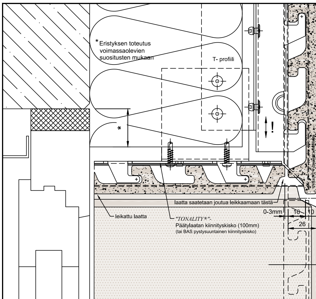
DETALJI "11.3" Nro. ADS 100-13
